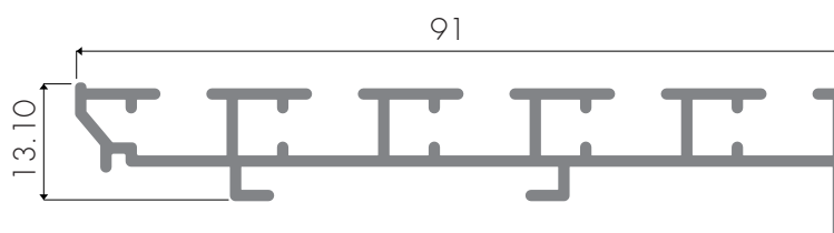
Riel 5 vías
