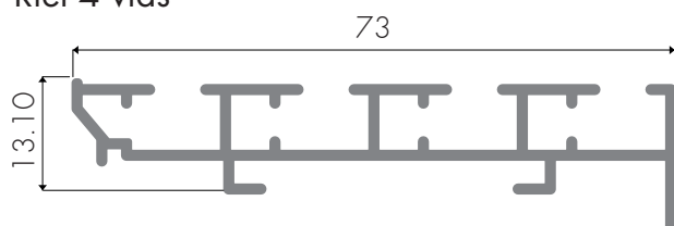
Riel 4 vías
