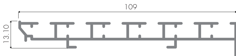
Riel 6 vías
