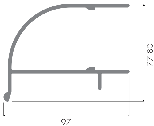
Riel techo
