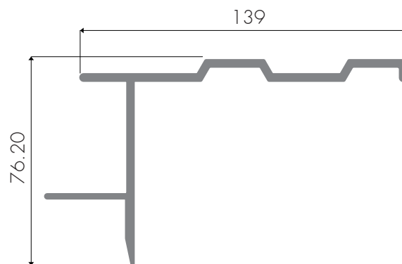
Larguero
